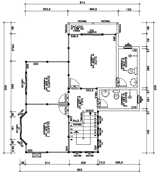
PAVIMENTO SUPERIOR A: 57,05 m 2
